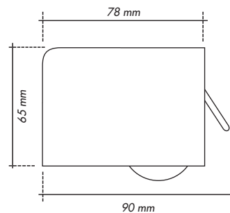
ruota Ø 50 con cuscinetto a sfera wheel Ø 50 with ball bearing
