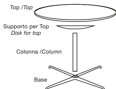
Componenti base Tavolo Components for Table
