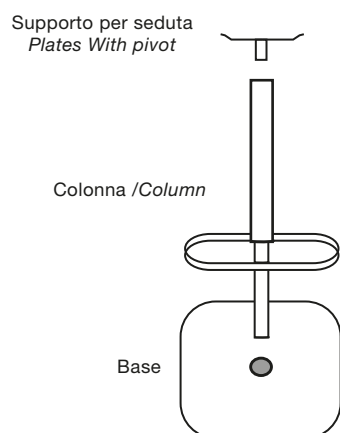
Componenti per Sgabello Components for Stool
