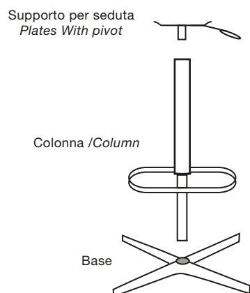
Componenti per Sgabello Components for Stool
